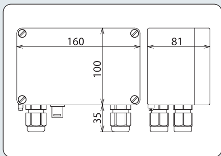
Размерный эскиз ИТАК EXI BXT
