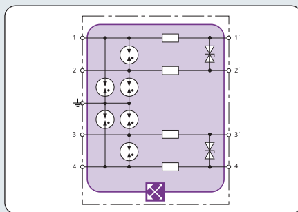
Принципиальная схема ИТАК EXI BXT
