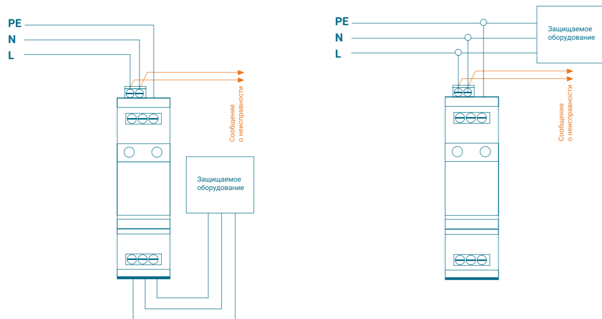
Последовательная установка РИФ-Э-III 320/3 с (1+1) в электрическую сеть.
