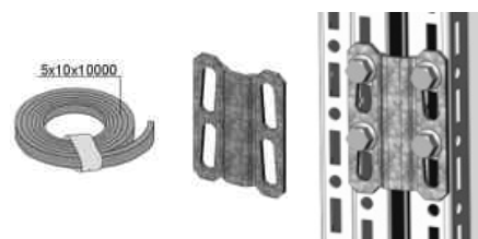
Комплект соединительный
