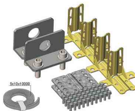
Комплект транспортировочный
